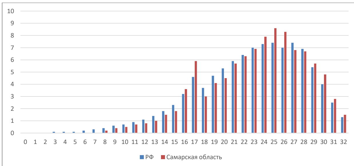
Диаграмма 2.1.3 Распределение первичных баллов
