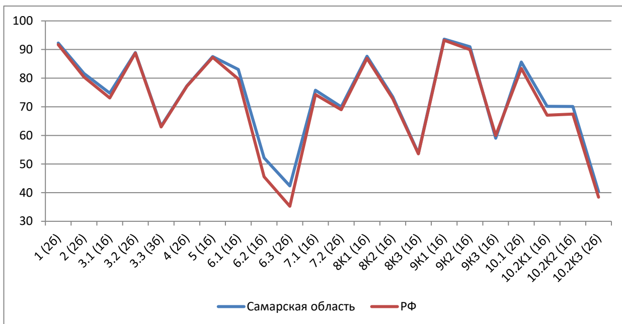
Диаграмма 2.1.4. Выполнение заданий
