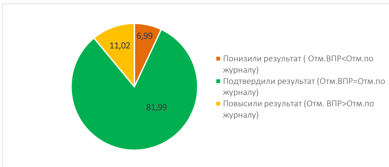
Диаграмма 2.1.2. Сравнение отметок с отметками по журналу
