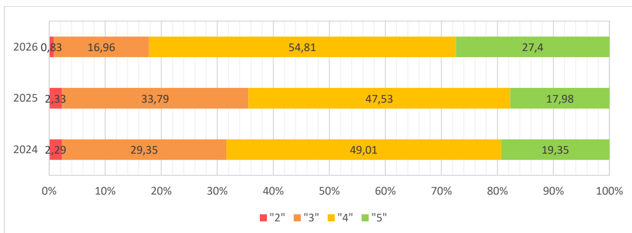
Диаграмма 2.1.1. Статистика по отметкам
